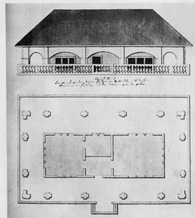
Защитный футляр для Домика Петра I. Чертеж из Стокгольмской коллекции
